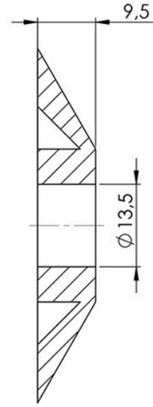
KESİT A-A
