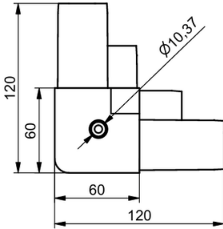
ÖN GÖRÜNÜŞ
