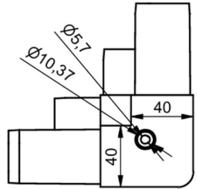
YAN GÖRÜNÜŞ
