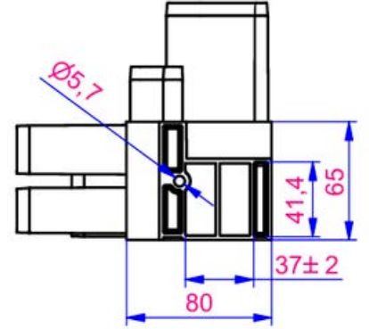
YAN GÖRÜNÜŞÜ
