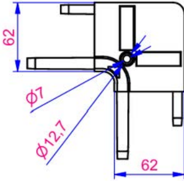
TABAN GÖRÜNÜŞÜ
