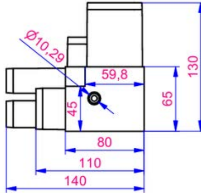
ÖN GÖRÜNÜŞÜ
