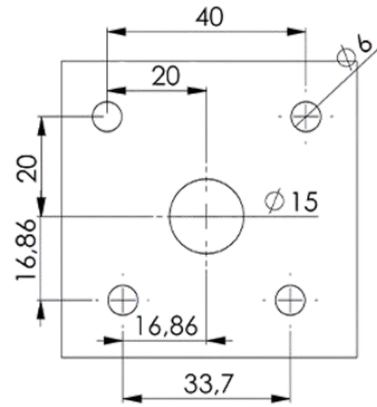
KAPI KOLU BAĞLANTI DETAYI
