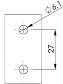
SABİTLEME PARÇASI BAĞLANTI DETAYI
