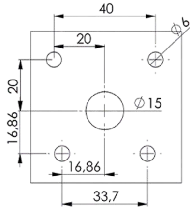
KAPI KOLU BAĞLANTI DETAYI
