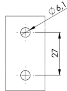
SABİTLEME PARÇASI BAĞLANTI DETAYI
