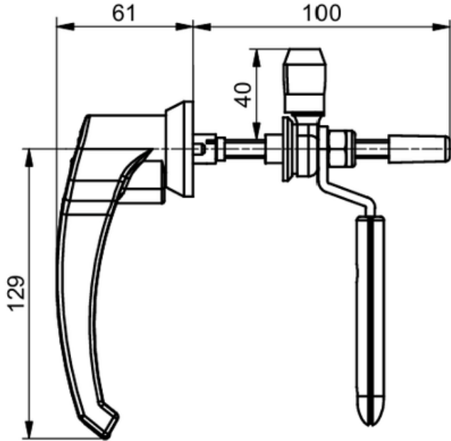
ÖN GÖRÜNÜŞ
